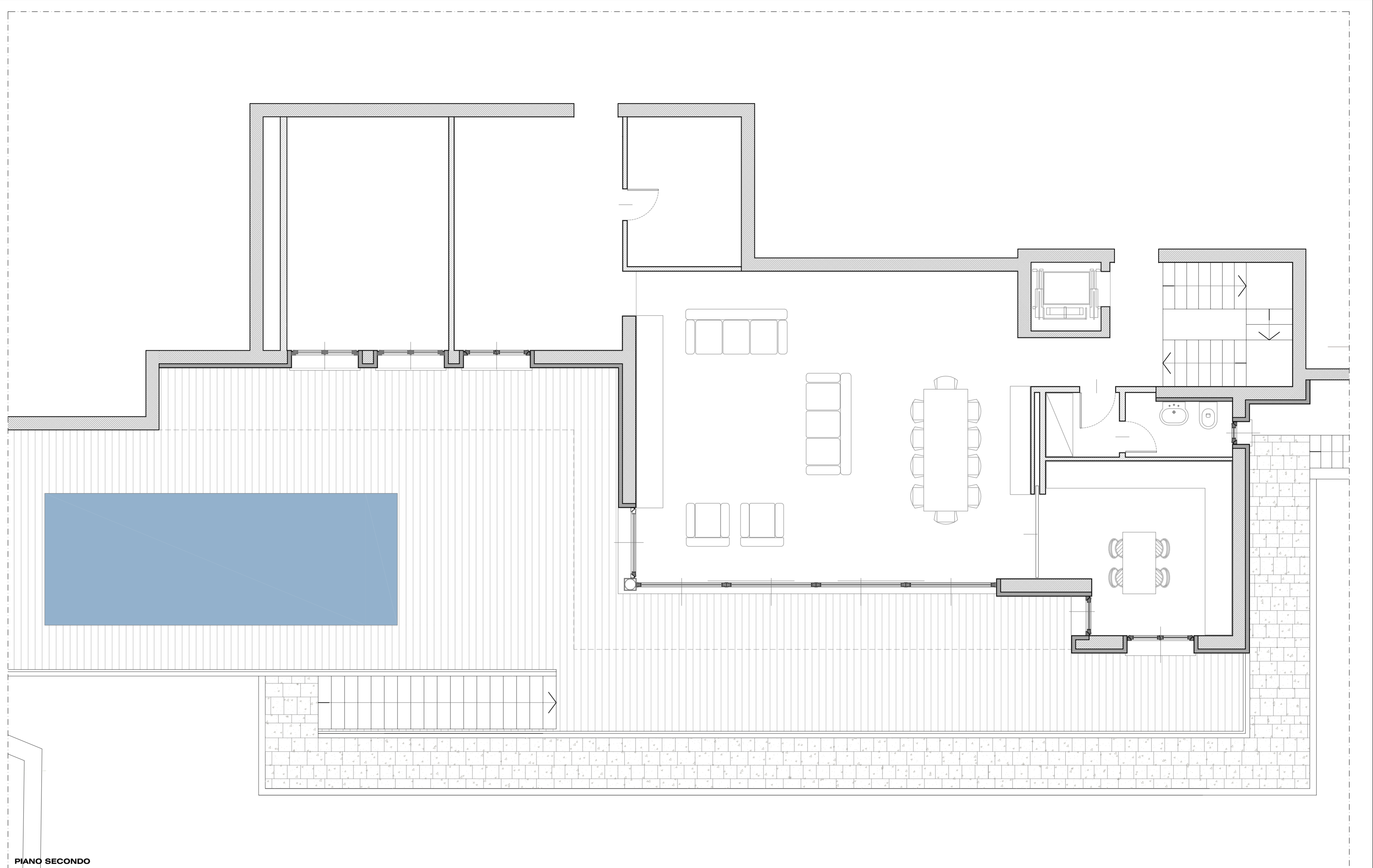
PIANO SECONDO
